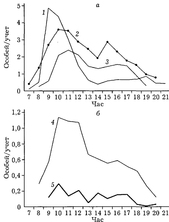
Рис. 2. Зависимость активности сирфид некоторых родов и видов от времени суток. а: 1 – Chrysotoxum , 2 – Helophilus , 3 – Cheilosia ; б: 4 – Myiathropa florea , 5 – Eupeodes .
